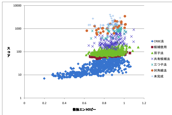
図 27 数独エントロピーとスコアの関係. Fig. 27 D -Score and SUDOKU entropy H_G .
