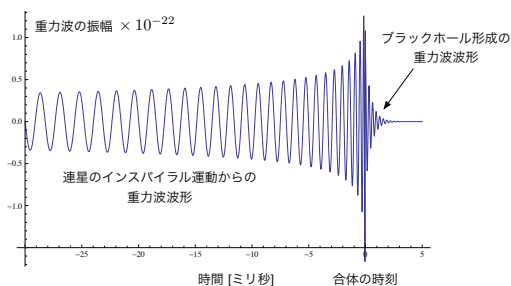
図6: 中性子星あるいはブラックホール連星の合体の前後で放出される重力波の波形(予想)。次第に振幅を大きくしながら、1kHzに近い周波数にまで上がる。合体後にブラックホールが形成されるならば、重力波はブラックホールに飲み込まれてしまい、急速に減衰する。この減衰部分が観測されれば、ブラックホールを直接観測したことになる。
