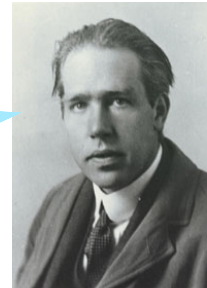
ボーア (コペンハーゲン解釈)
