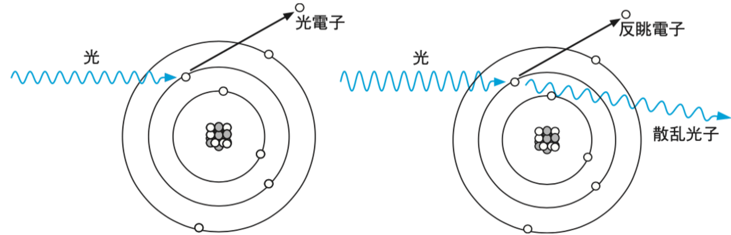
図 4.21 [左] 光電効果. [右] コンプトン効果. どちらも光を当てると電子が飛び出す現象であるが, コンプトン効果は, 光のエネルギーが大きくて, 軌道電子にエネルギーが完全に吸収されないときに見られるようになる.
