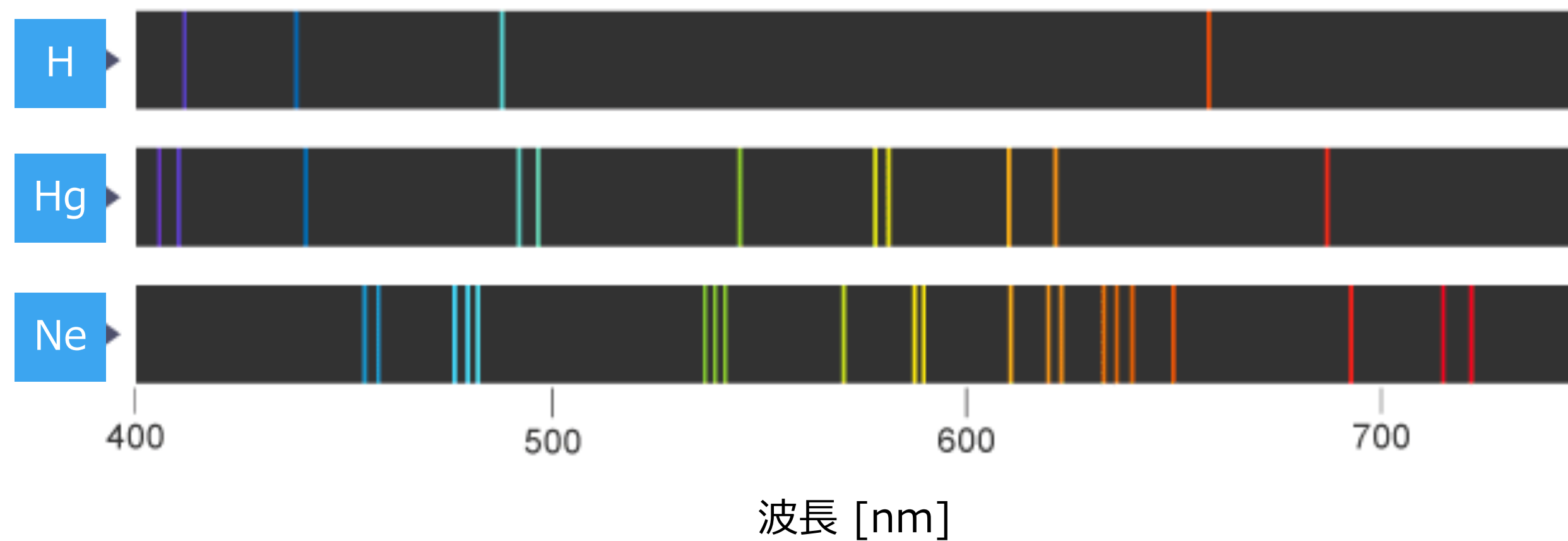
(a) 元素が放つ輝線スペクトル
