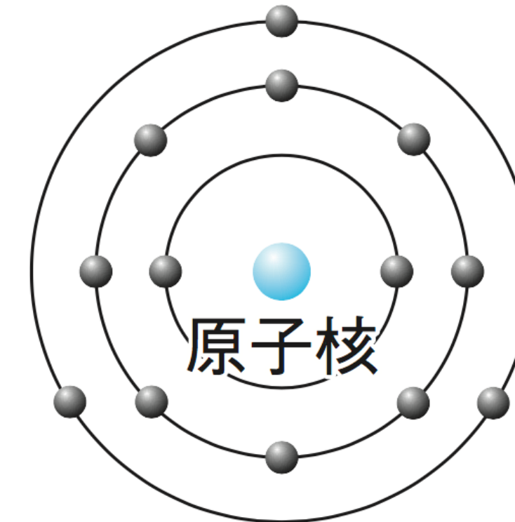
ラザフォードの 原子模型
