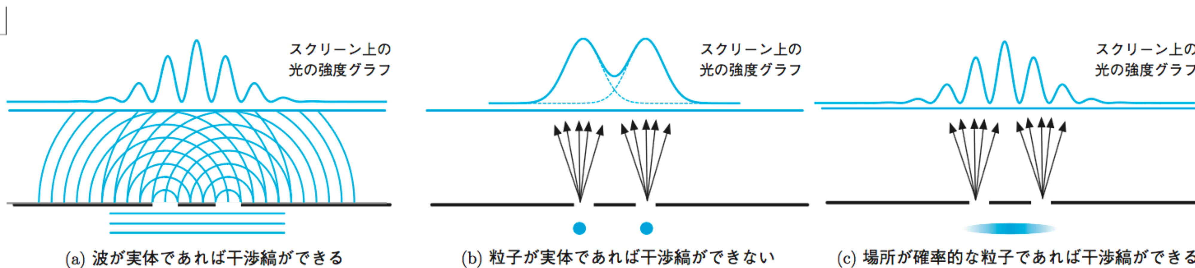
図 4.27 コペンハーゲン解釈による 2 重スリット問題の解釈. 光が粒子であれば干渉縞が生じないはずだが, 実際には干渉縞が生じている. そこで, 粒子ではあるが, ミクロの世界では, 確率的にしか場所が特定できないもの, と考える.
