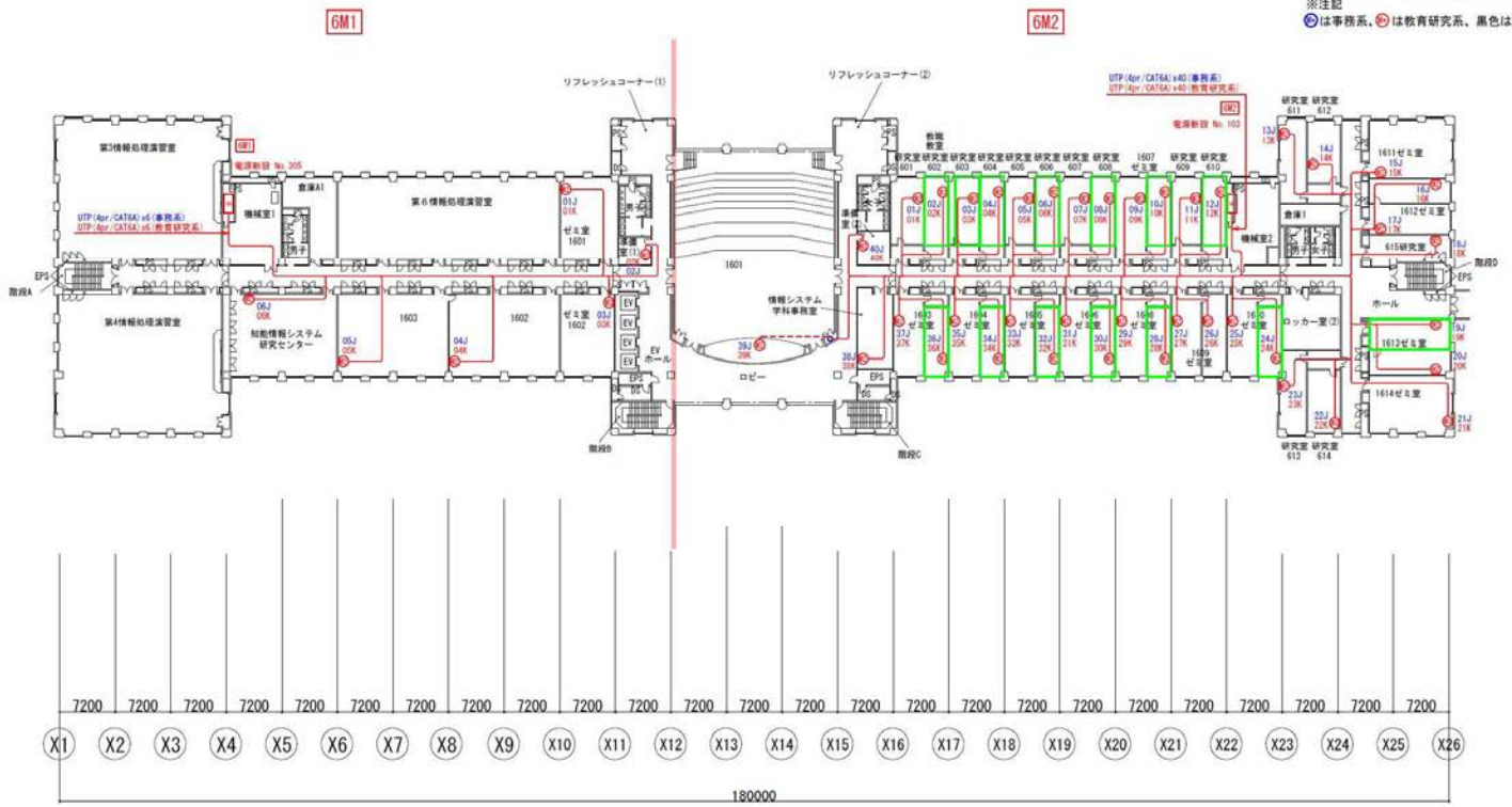
6階平面図
