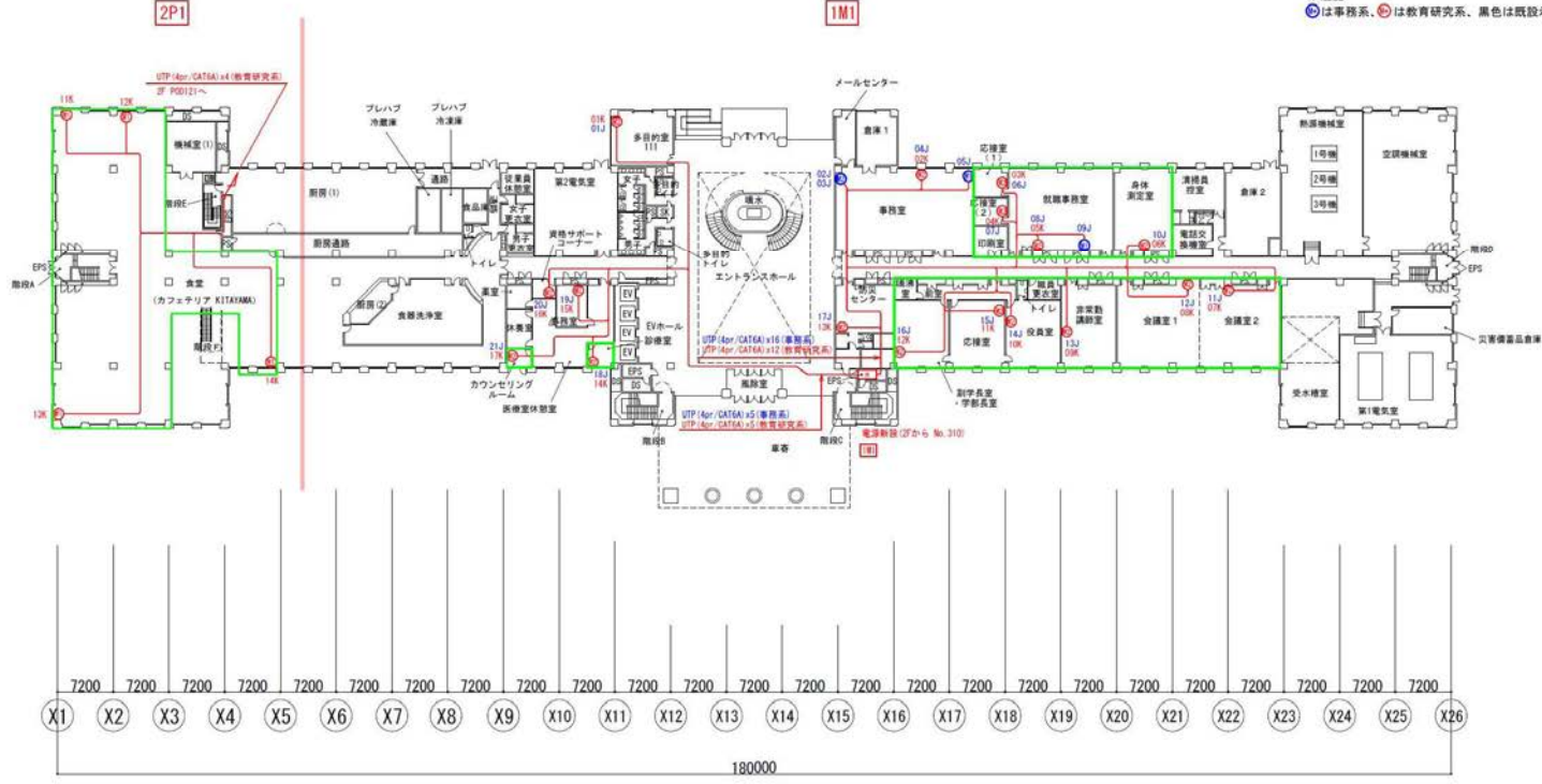
1階平面図
