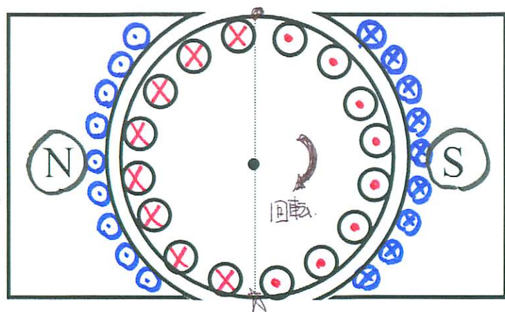
発電機 の補償巻線
