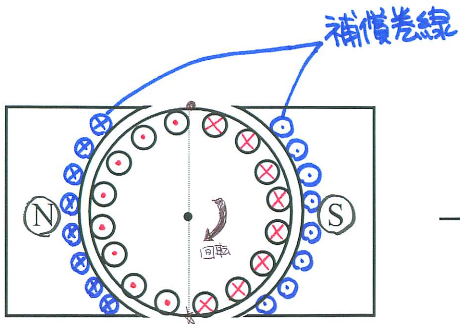
電動機 の補償巻線
