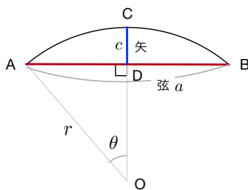
図 4.2: 『九章算術』の弧田問題 (方田の第 35・36 問).
