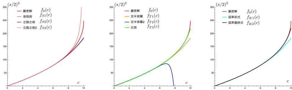
図 A.1: 建部の導いた半背の2乗の値を厳密な値と比較したもの. 横軸は矢の長さ c で, c = 10 は半径と一致する場合 ( \pi/2 の場合) である.
