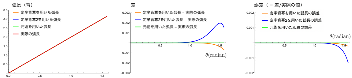
図 4.5: 弧長を建部の展開式から導出したもの。横軸は角度 (radian) で \pi/2 まで。
