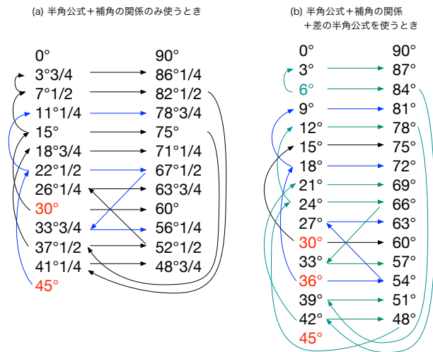
図 3.4: 60^\circ と 90^\circ の正弦と, 補角の関係, 半角の公式が既知であれば, 24 の角度の値での数表が作成できる (図 3.2 と原理は同じ). さらに差の半分の正弦を求める公式 (20) が既知であれば, 30 の角度での数表が作成できる. 右図は, 27^\circ と 15^\circ の正弦から 6^\circ の正弦を求めたときの例.
