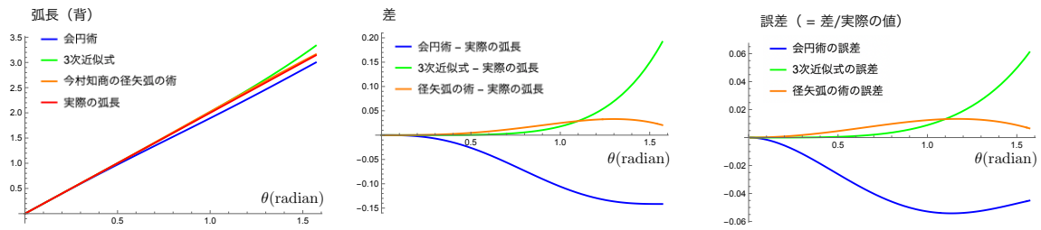
図 4.4: 『会円術』の弧長 (35) と 3 次近似式 (37) を実際の弧長と比較したもの。今村知商『豎亥録』径矢弦の術による弧長も示す。横軸は角度 (radian) で \pi/2 まで。
