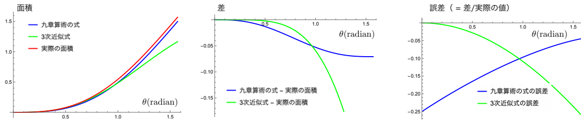
図 4.3: 『九章算術』の弧田面積式 (30) と 3 次近似式 (34) を実際の面積と比較したもの．半径 1 の円を想定した．横軸は角度 (radian) で \pi/2 まで．
