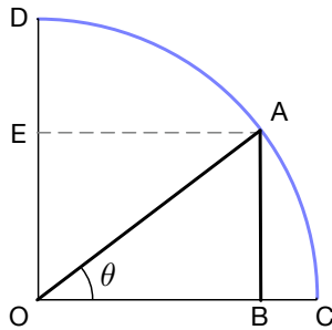
図 3.5: パースカラ 2 世による 4 つの三角関数の定義. Figure 3.5: Definition of the four trigonometric functions by Bhaskara II.
