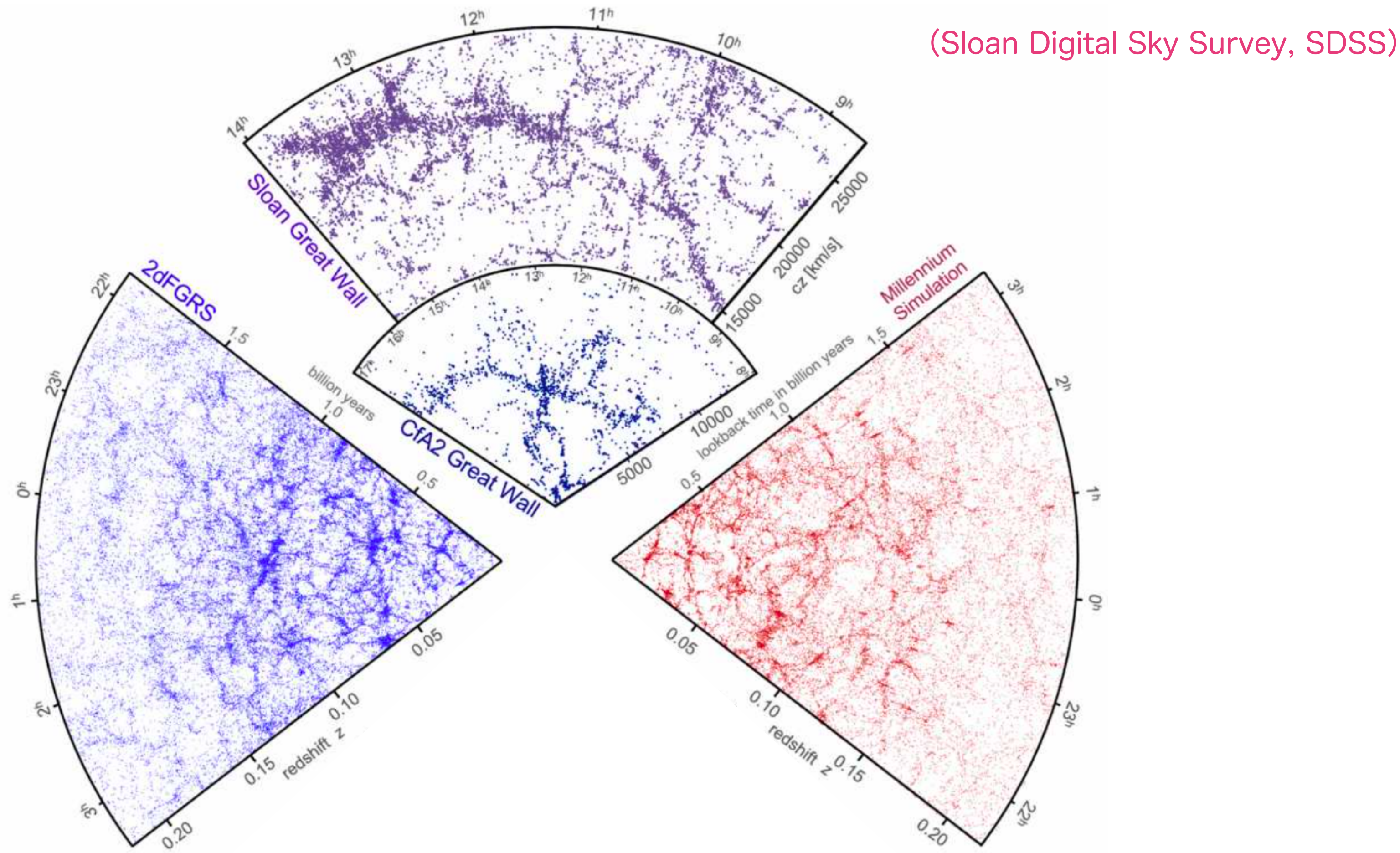
図 1.35 銀河の分布観測とシミュレーションによる疑似分布を並べたもの。〔上〕SDSS サーベイによる銀河の分布図と図 1.34 を重ねたもの。SDSS は、北天から見える 65 万個以上の銀河を 2 億光年まで示している。1.3 億光年の距離に及ぶ 1 万個以上のグレートウォール（万里の長城）も新たに発見された。〔左〕2dFGR サーベイによる銀河の分布図。南天の 22 万個以上の銀河を 2 億光年まで示している。〔右〕ミレニアム・シミュレーションという数値計算結果を似せて示したもの。[Springel, Frenk, White の論文 (2006) を加工]
