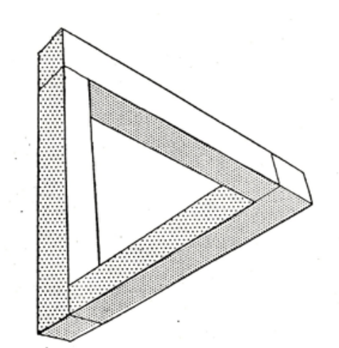
不可能立体の一つ「ペンローズの三角形」
