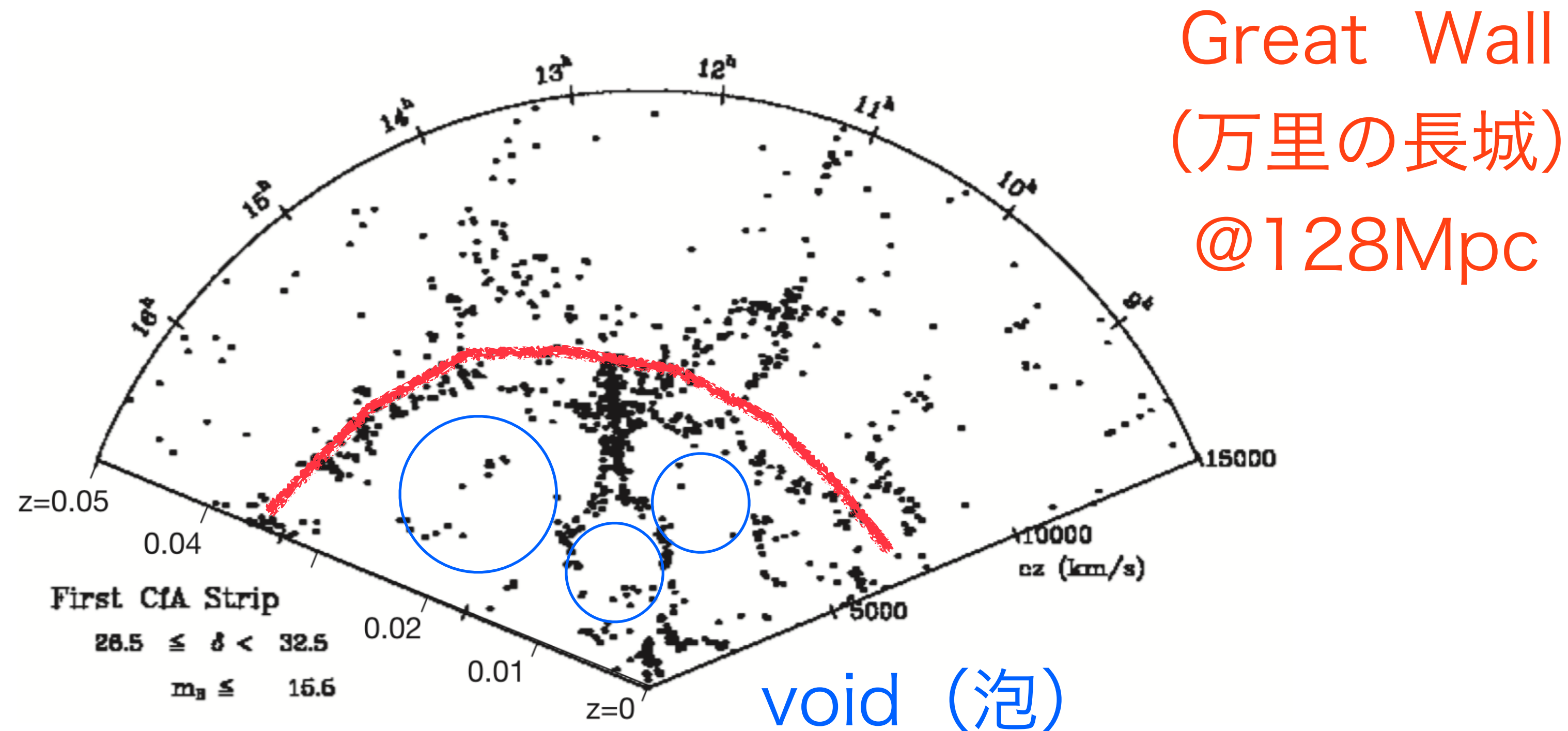
図 1.34 1989 年に報告された CfA サーベイの図. 扇子を広げたように, 見かけの範囲を狭く, 奥を深く銀河をサーベイした結果の図である. 中心はかみのけ座銀河団 (Coma cluster). 1 つ 1 つの点が銀河であり, 全部で 1027 個のデータがある. 右側の距離の目盛りは赤方偏移から測った後退速度を示している. 左側の目盛りは赤方偏移 z を記入した. z = 0.03 と記された距離が 128 Mpc に相当する. [CfA が提供している図を加工]
