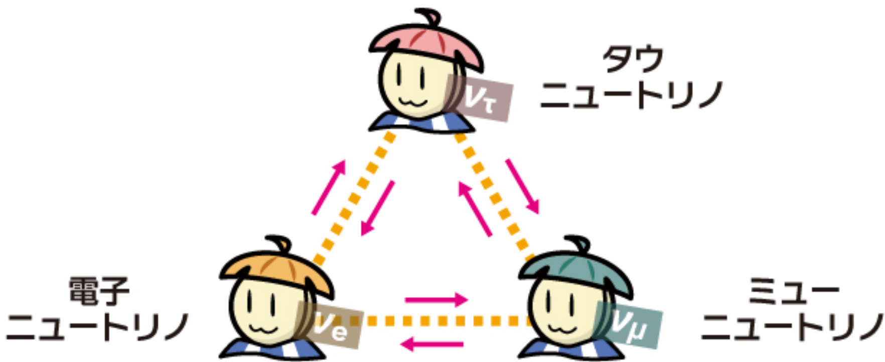
各ニュートリノの間で入れ替わる確率
