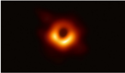
日米欧の研究チームが2019年4月に発表した、M87銀河のブラックホールの画像。黒い穴の部分がブラックホール=EHT collaboration
