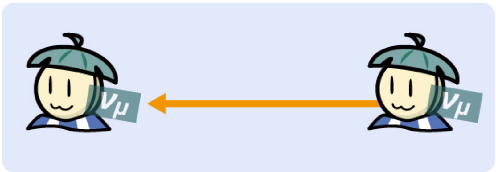
ニュートリノの移動した距離
