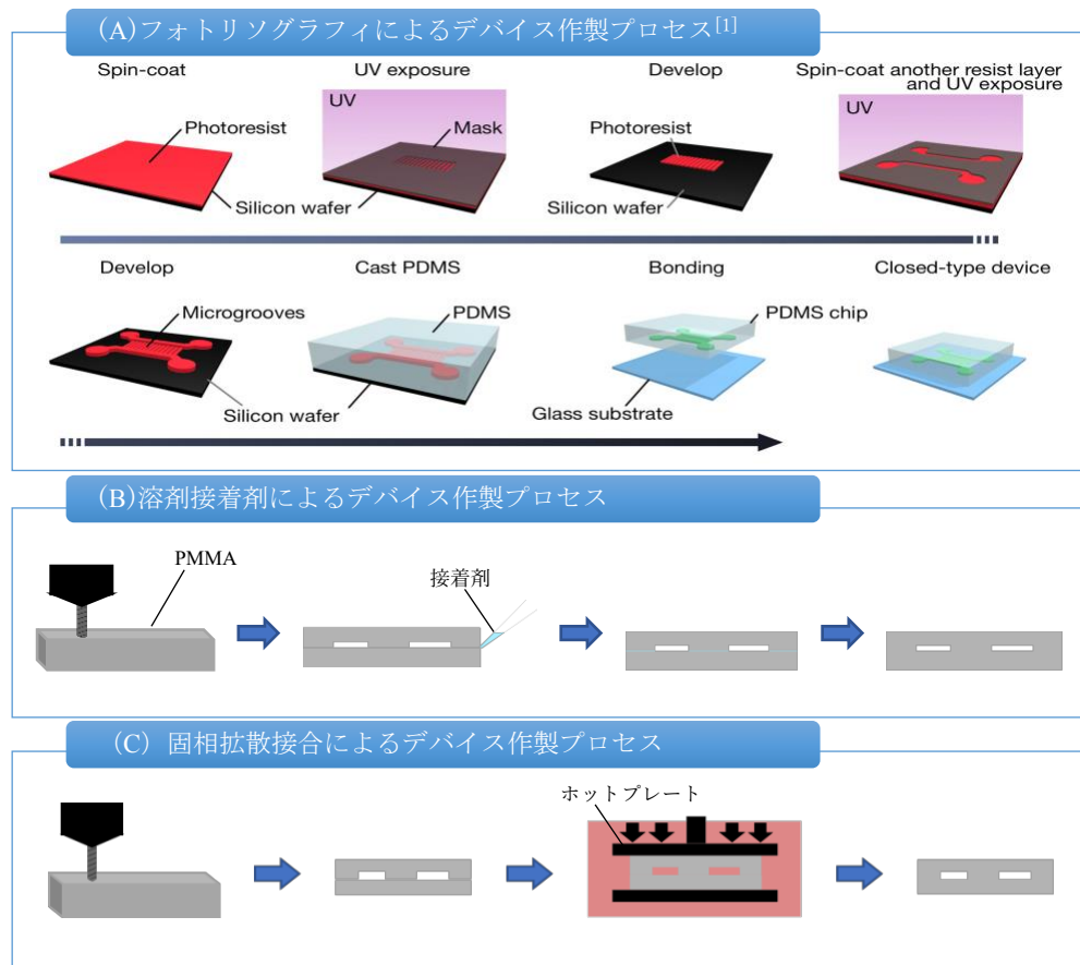
図1 マイクロ流体デバイス作製プロセス：PDMSとPMMAを比較。(A) フォトリソグラフィによるデバイス作製プロセス [1] 。デバイス完成までの所要時間は約2週間～を要し、費用は約2000万円である。(B) 接着剤によるデバイス作製プロセス。デバイス完成までの所要時間は約0.5時間～を要し、費用は約50万円である。(C) 固相拡散接合によるデバイス作製プロセス。デバイス完成までの所要時間は約1.5時間～を要し、費用は約300万円である。
