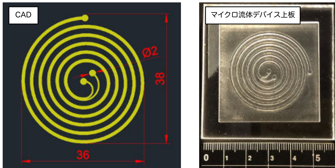
図6 PMMA製分離用マイクロ流体デバイス
