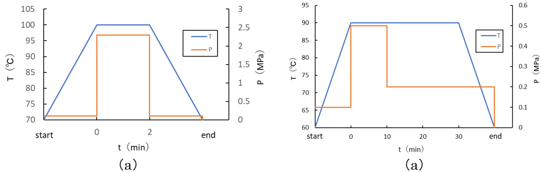
図3 固相拡散接合の一例 (a) 100 °C、2.3 MPaで2分保持。(b) 90 °C、0.5 MPaで10分保持したのち、0.2 MPaに減圧し20分保持。
