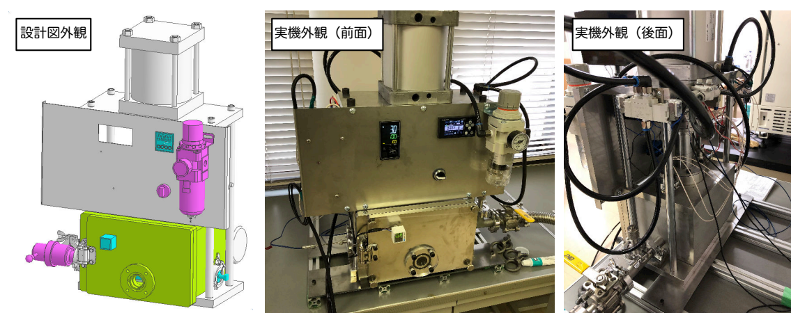
図2 設計・開発した固相拡散接合装置
