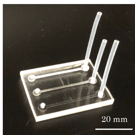
図5 通水試験用マイクロ流体デバイス
