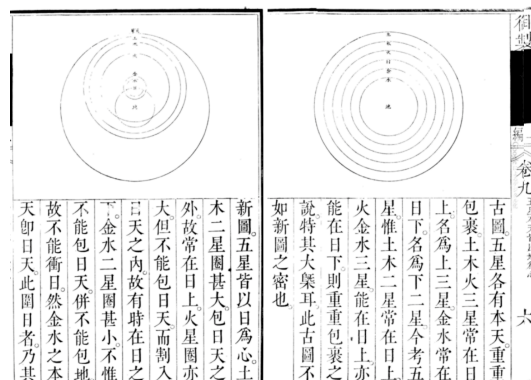
図 2: 『曆象考成 五星本天皆以地為心』にある古図と新図。天動説とティコ(第谷)の説が紹介されている。(https://books.google.co.jp/より)
