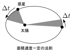
図 1: 面積速度一定の法則
